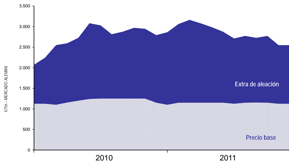
Precios de chapa de acero inoxidable | AISI 304 laminada en frío 2,0mm 2010-2011
