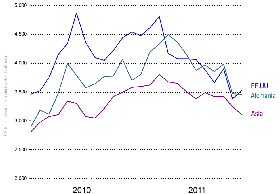
Precios de chapa de acero inoxidable | AISI 304 laminada en frío 2,0mm 2010-2011
